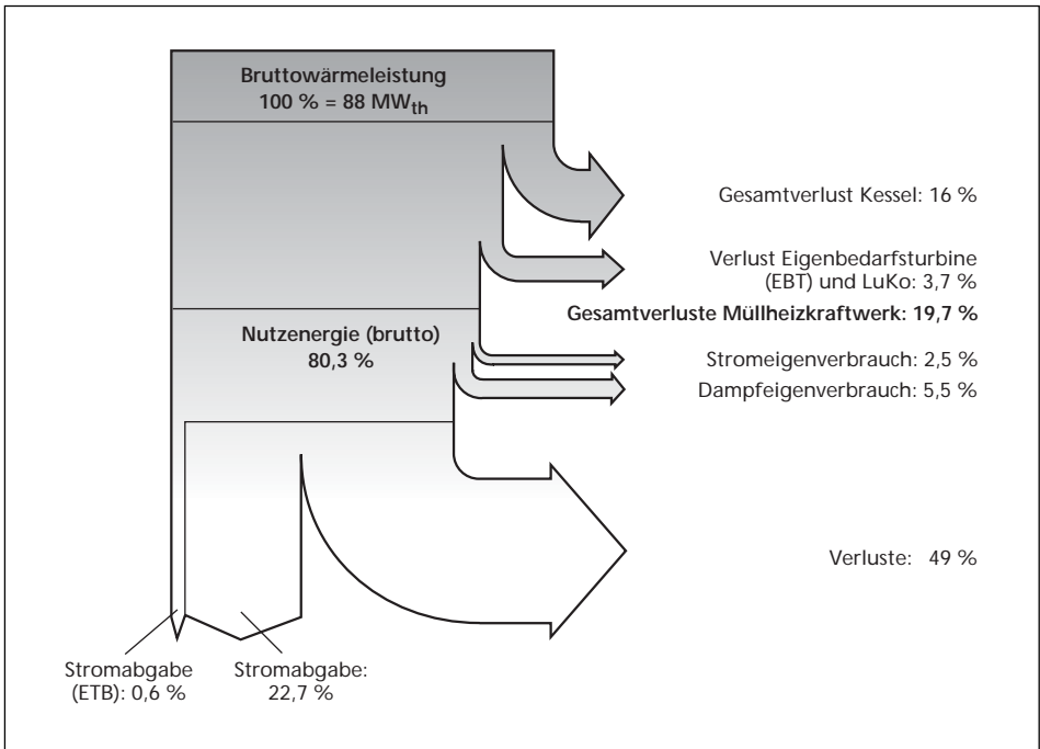
Bild 4: Energieabgabe und -verluste des MHKW Mainz bei stromoptimierter Fahrweise
