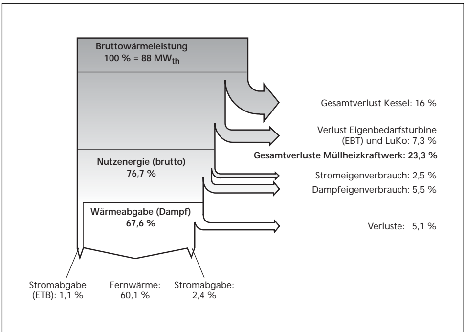
Bild 5: Energieabgabe und -verluste des MHKW Mainz bei wärmeoptimierter Fahrweise
